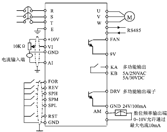
下图为HLP-CP出厂时标准配线图
