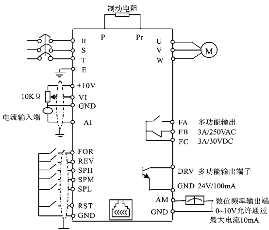
下图为HLP-CP出厂时标准配线图
